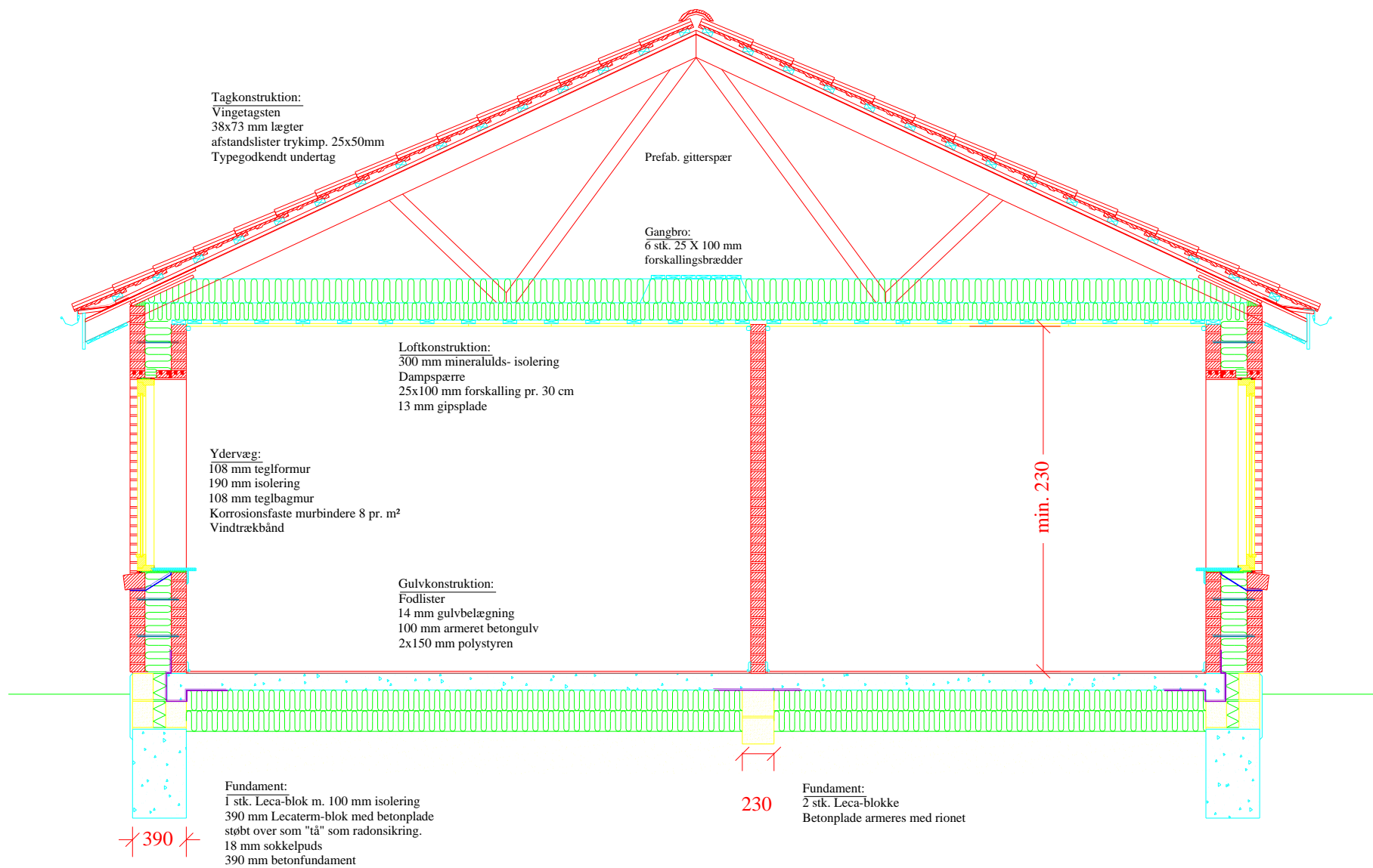
Tværsnit 1:50
