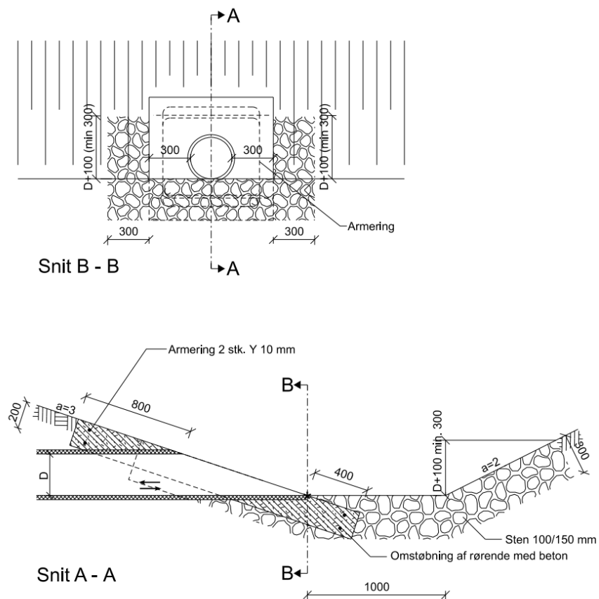
Figur 1 Principskitse af tværsnit af udløbsbygværk.
