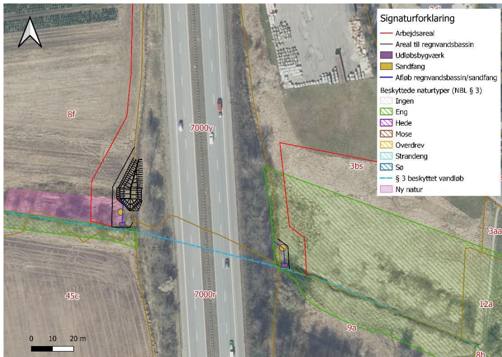
Figur 2 Oversigt over etablering af grøftebassin og udløbspunkter langs Motorvej E45 nord for Svejstrup Bæk.
