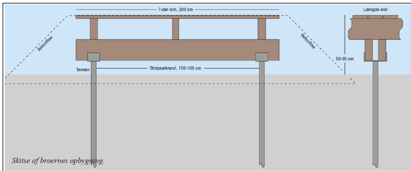
Figur 4 – Principskitse af broernes opbygning. Skitsen er fra ansøgningsmaterialet.
