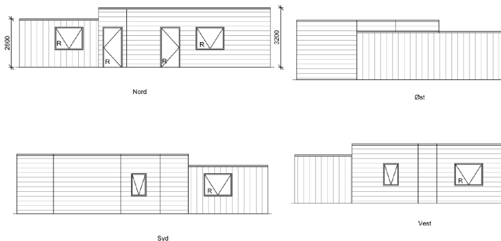
Figur 1 Opstalter
