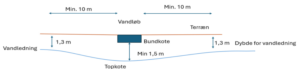
Figur 1 Principskitse for vandløbskrydsning for vandledninger
