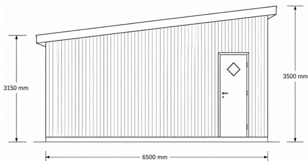
Figur 3 Facade mod nord
