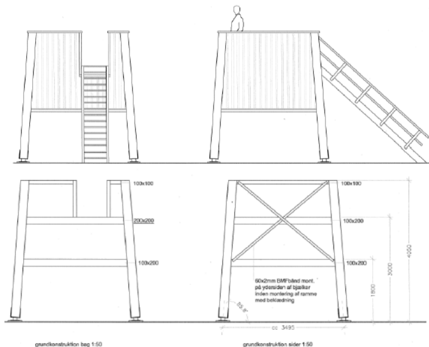
Billede 1: Skitse af udkigstårn.
