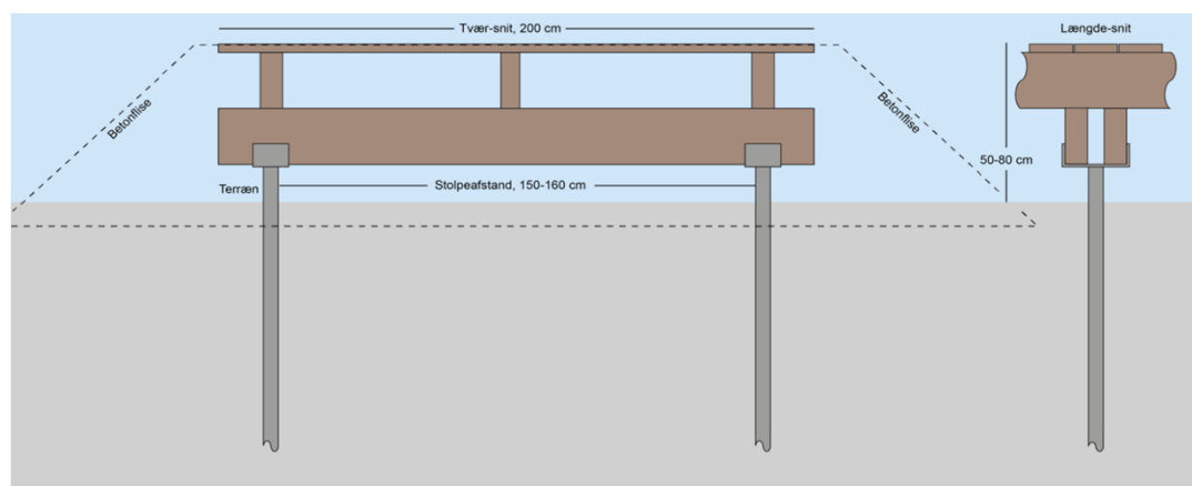
Figur 4 – Principskitse af træstierne. Bemærk at der er luft under de langsgående vanger, svarende til mindst højden af det træ som de langsgående vanger hviler på, mindst 25 cm.
