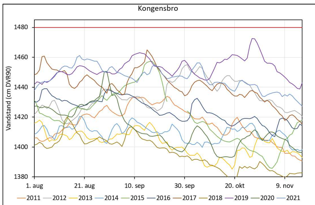
Figur 4-4 Opstrøms Tange Sø. Udløsende kontrolvandspejl på kontrolstation Kongensbro (rød linje) samt døgnmiddelvandstand i årene 2011 – 2021.
